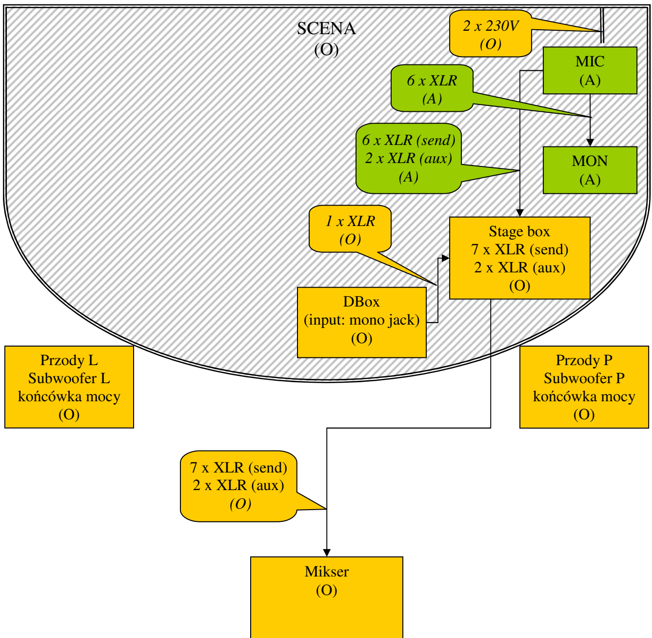
Rys. 2. Sprzęt nagłośnieniowy - wariant 2
