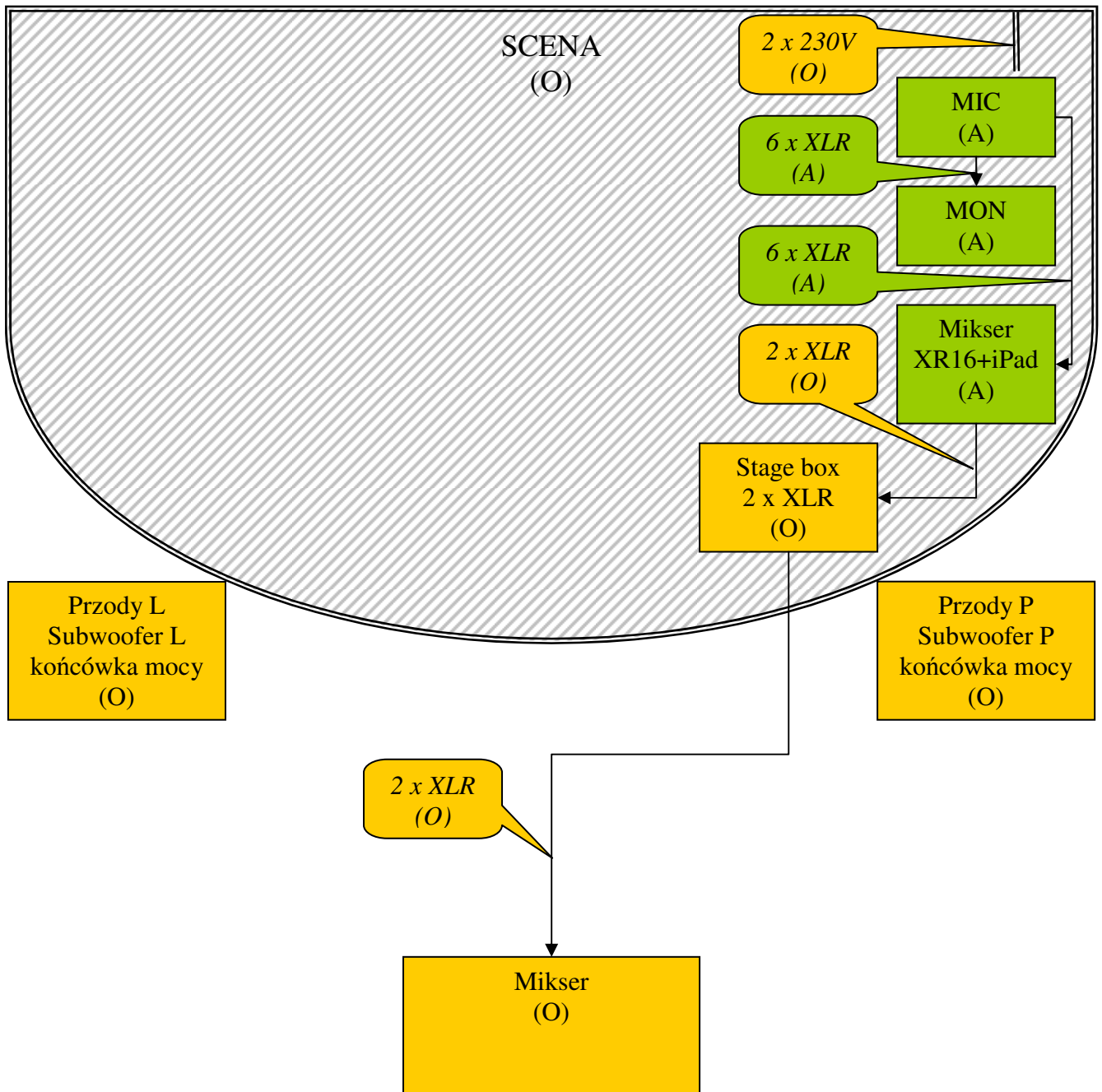
Rys. 1. Sprzęt nagłośnieniowy - wariant 1
